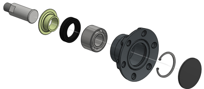
Roulement
